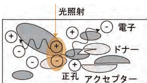
図1 有機薄膜太陽電池における光照射後の初期過程の概略図
