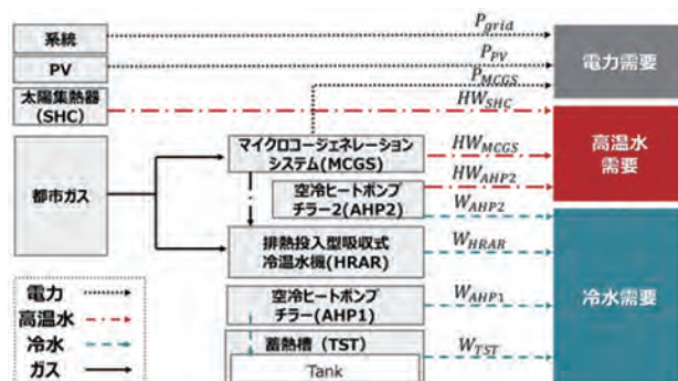
図2 U市庁舎の空調熱源フロー
