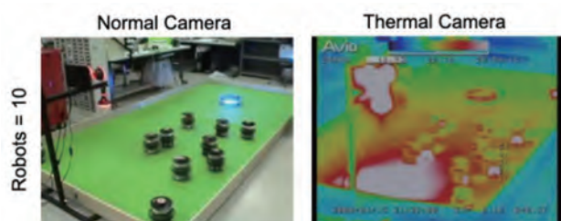
写真1 群ロボットによる協調運搬
