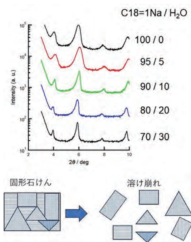
図1 (上) 水を含んだ石けんの小角X線回折 (下) 解明された石けんの溶け崩れ機構
