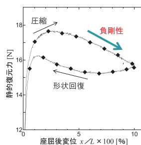
板状形状記憶合金の座屈変形時の負剛性特性と、この特性を利用したパッシブ除振機構の試作機
