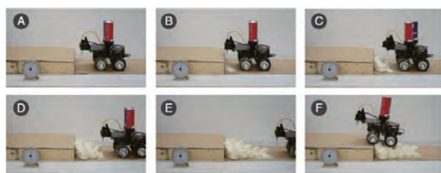
写真2 ロボットが発泡ウレタンを射出して段差を登る
