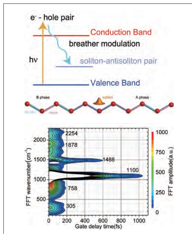
図2 trans-polyacetyleneの超高速分光 光励起後200fs以内でプレザソリトンと C-C、C=C伸縮振動モードが結合してサイトバンドが発生する。
