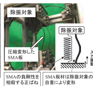
板状形状記憶合金の座屈変形時の負剛性特性と、この特性を利用したパッシブ除振機構の試作機
